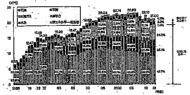
【図211-3-11】一次エネルギー国内供給及び電力化率の推移
